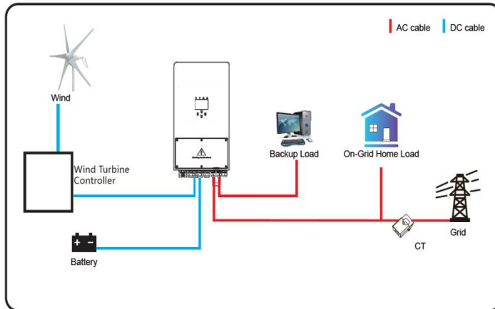
Modo II: Con microturbina eólica.
