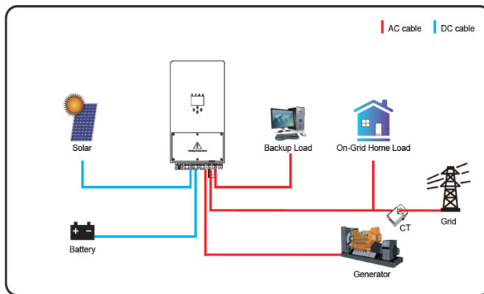
Modo IV: Con carga inteligente.
