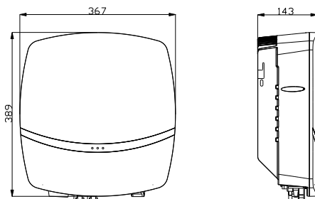
Figura 3.3 Dimensiones de R5-3K/3.6K/4K/5K/6K-S2
